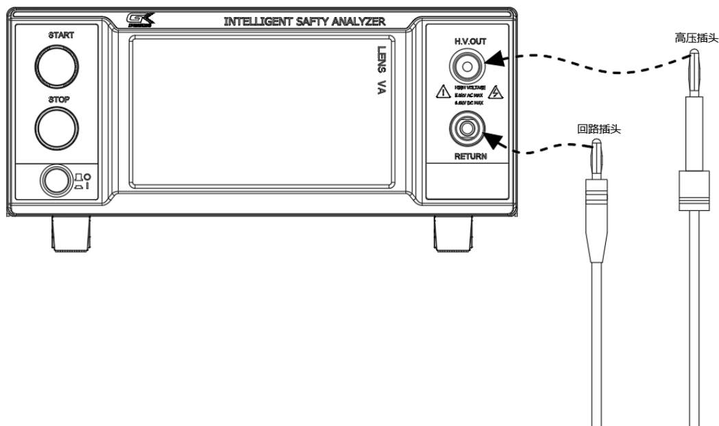
图 4-4-1 接线图
