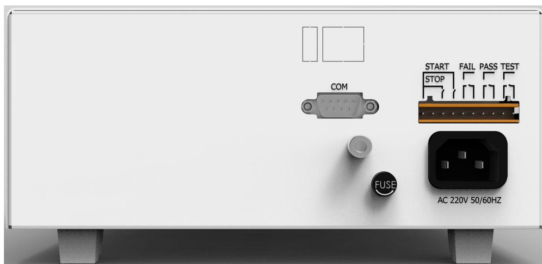
图 3-2-2 后面板
