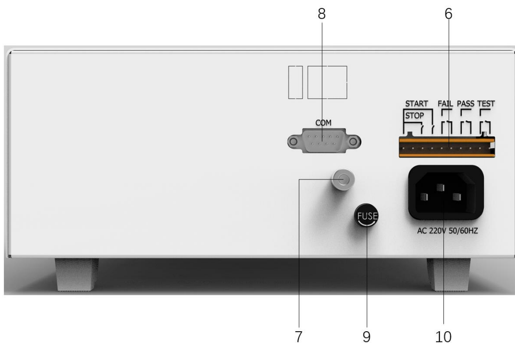
图 4-3-1 后面板
