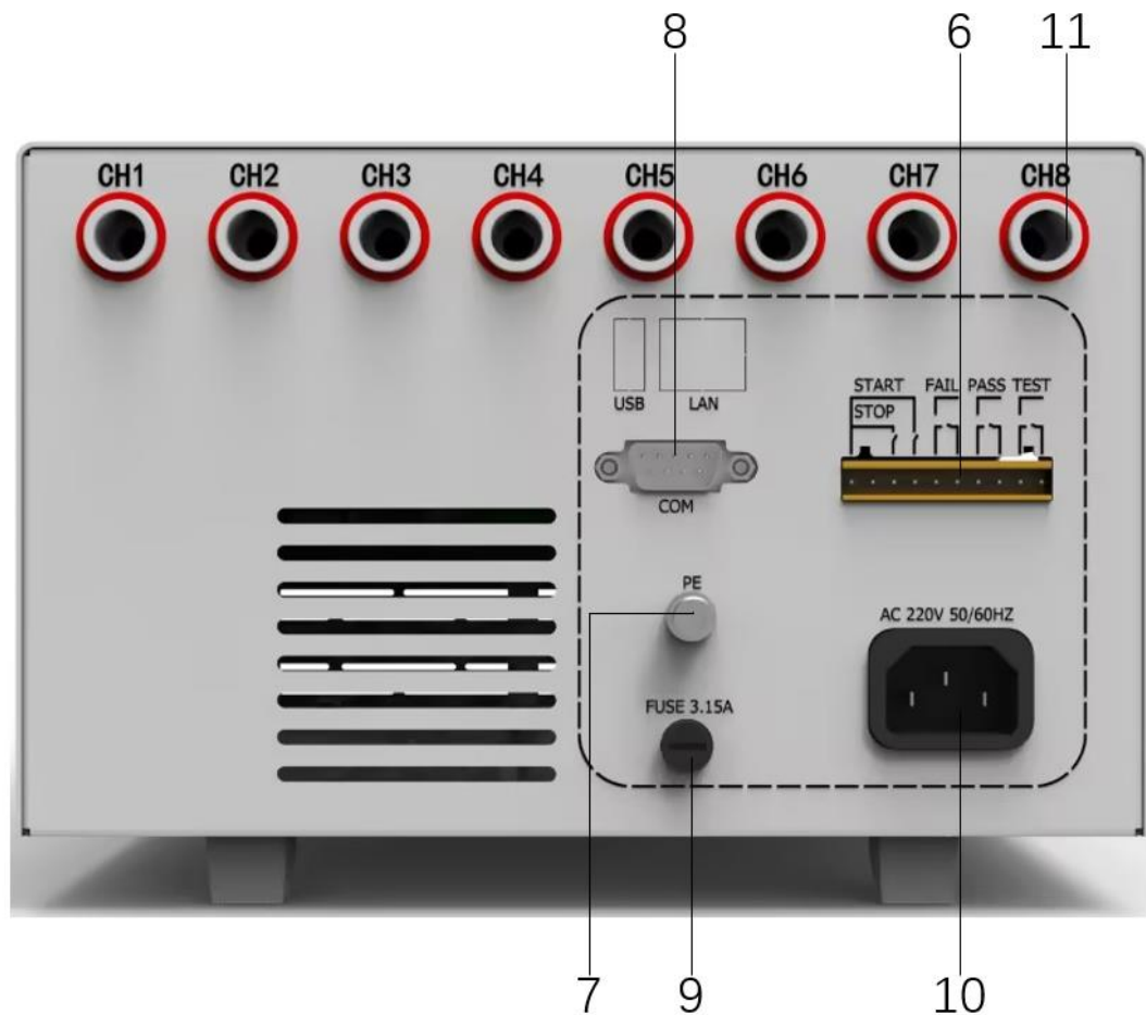
图 4-3-1 后面板
