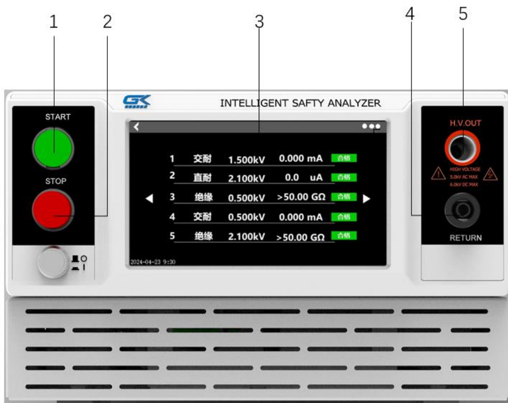
图 4-2-1 前面板
