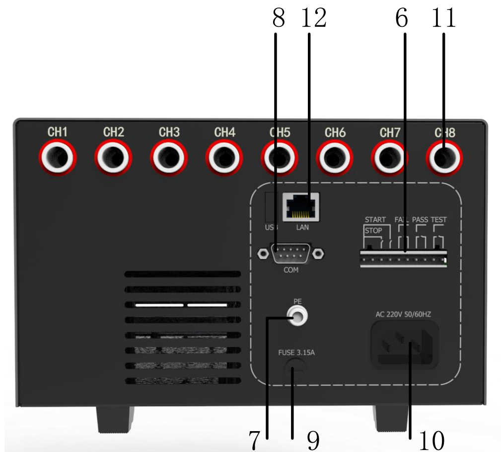
图 4-3-1 后面板
