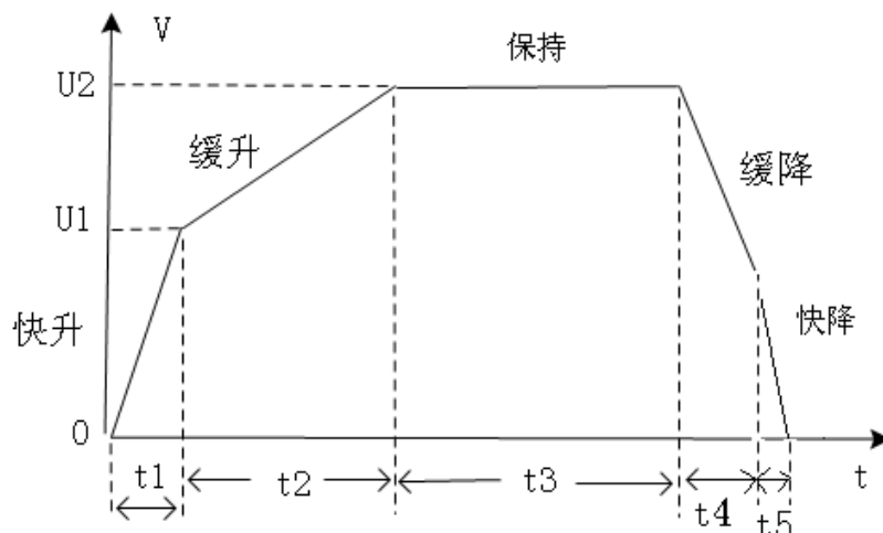
图 5-3-3 电压快升、缓升、保持、缓降和快降时间
