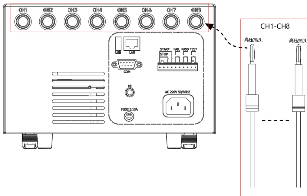
图 4-4-1 接线图
