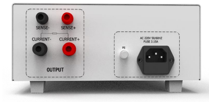
图 3-1-2 后面板
