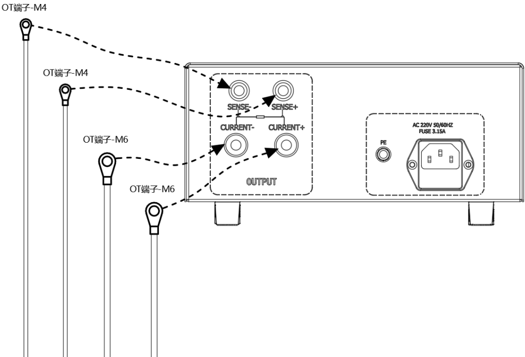
图 4-4-1 后面板
