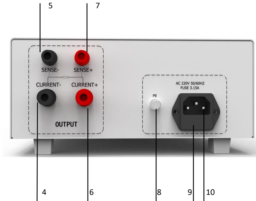
图 4-3-1 后面板
