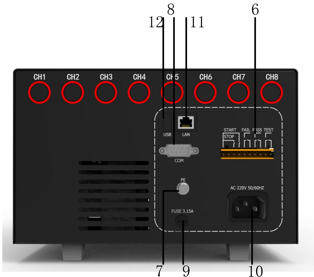
图 4-2-2 后面板
