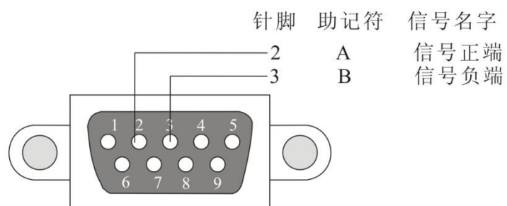
(b) RS485 接口信号定义
