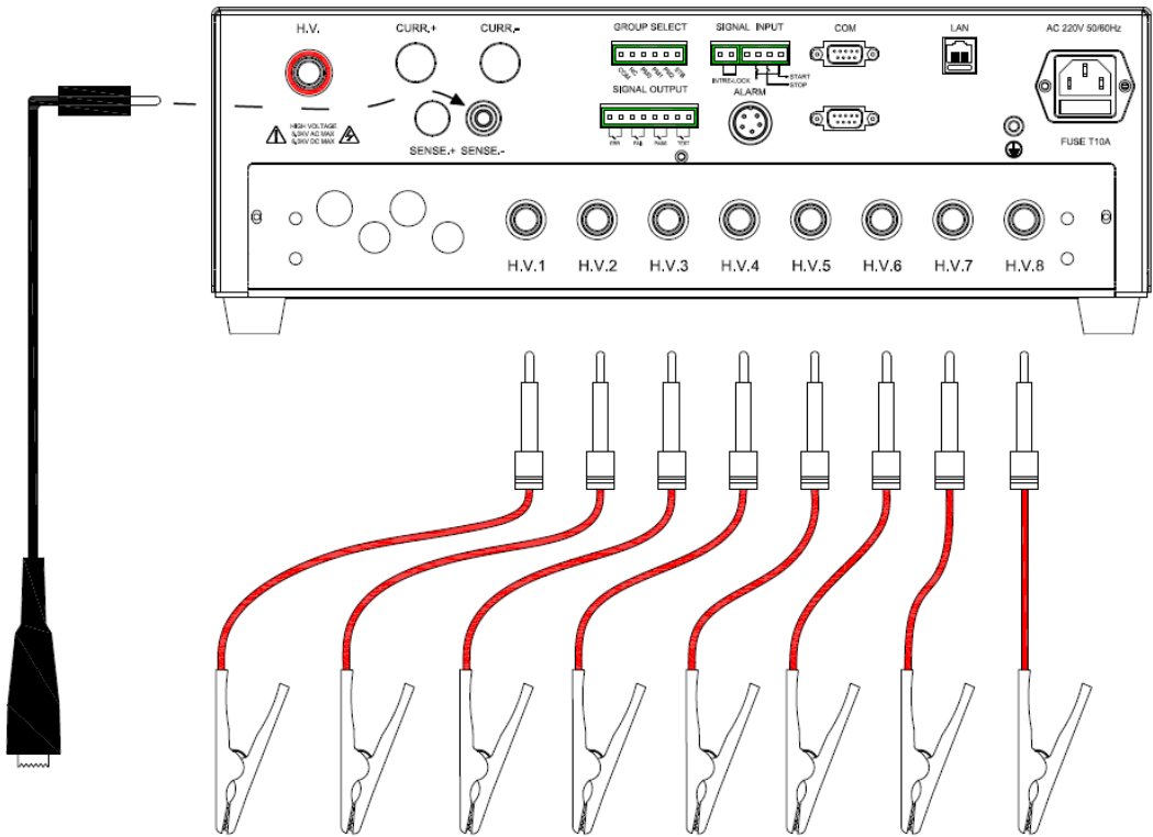
图 5-1-1 HEX301-8S 接线图
