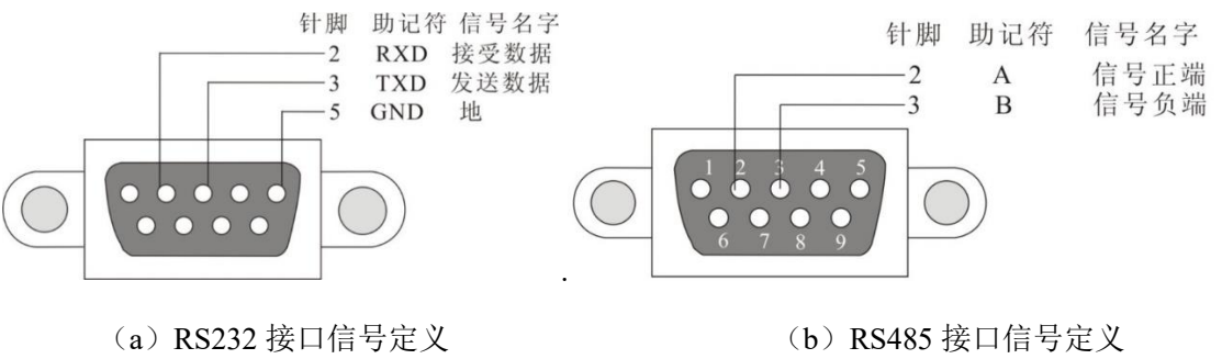
图 6-7-1 通信接口定义
