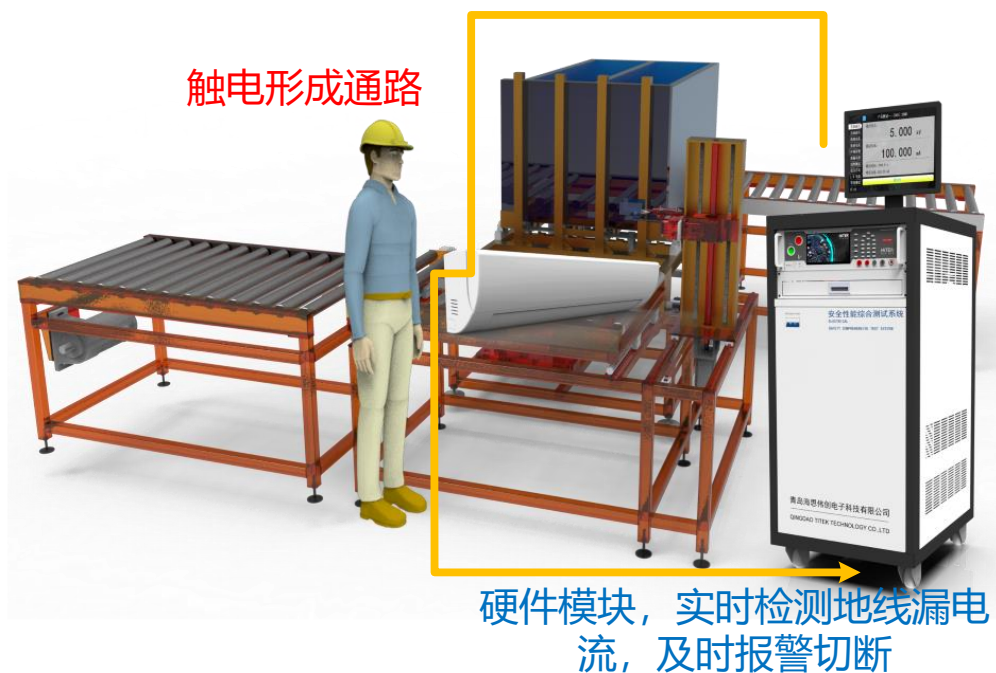
图 3-1-1 漏电快速断电保护原理
