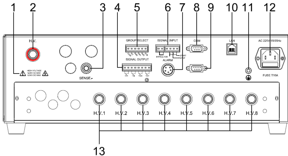
图 4-3-1 HEX301-8S 后面板说明
