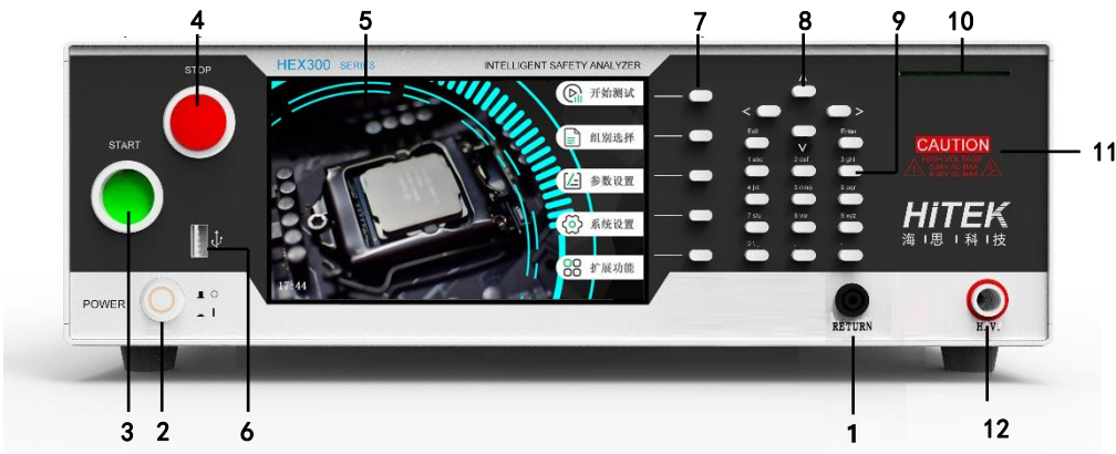
图 4-2-1 HEX301-8S 前面板说明
