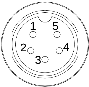
图 5-1-1 报警灯口插座（公）
