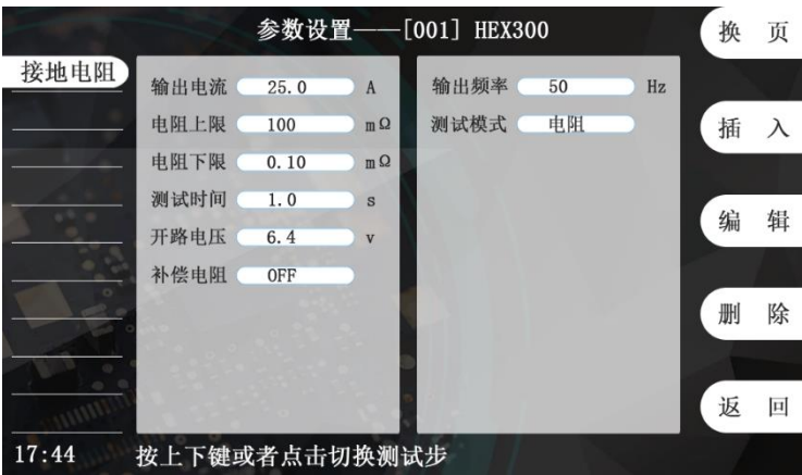
图 4-5-1 测试组设置界面
