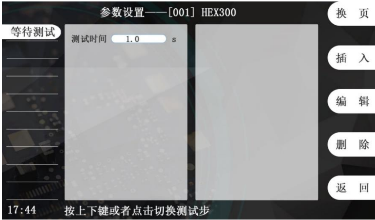
图 4-5-3 测试等待设置界面
