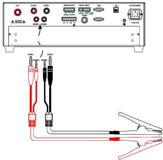
图 4-1-1 接地测试钳示意图
