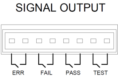
图 5-2-1 PLC 接口插座（公）
