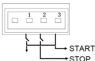
图 5-3-1 遥控口插座（公）
