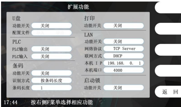
图 4-7-1 扩展功能界面
