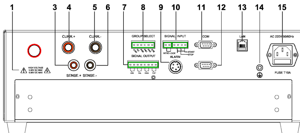
图 3-4-1 HEX303 背板说明
