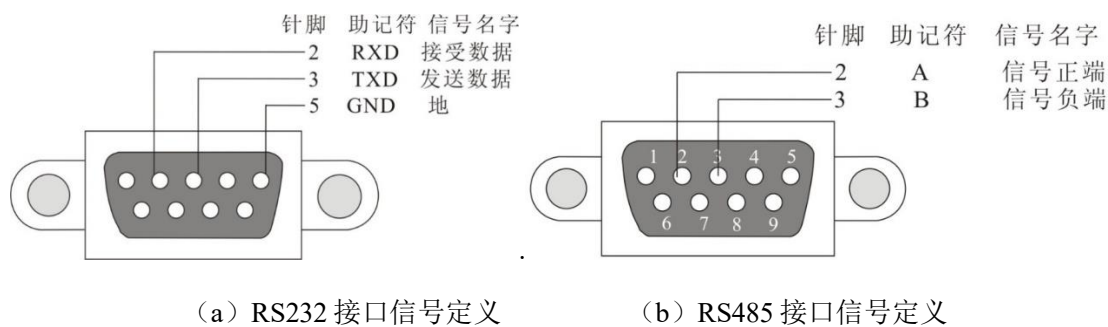
图 5-7-1 通信接口定义
