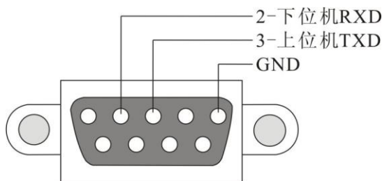
图 7-2 通信接口
