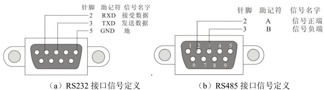
图 6-2-1 通信接口定义
