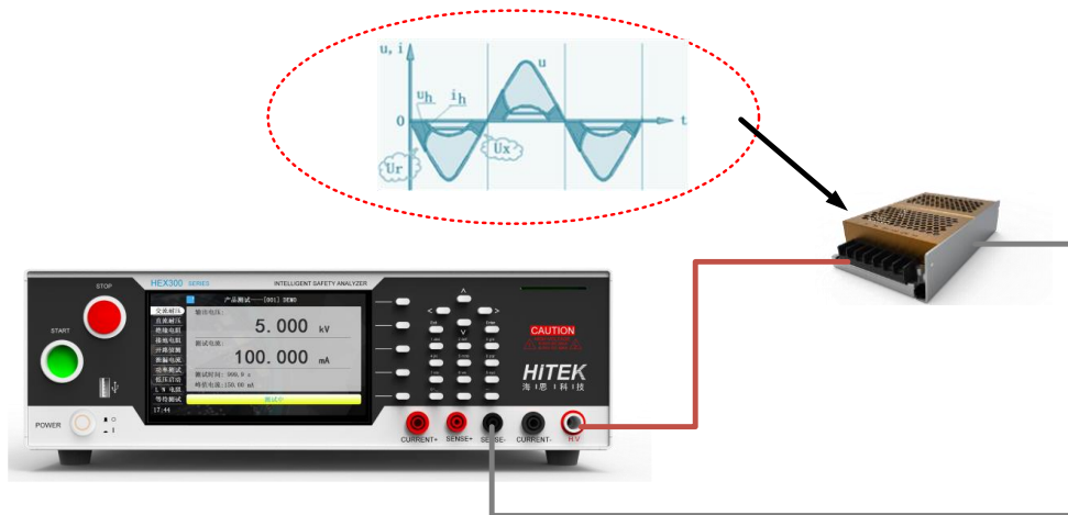
图 3-1-3 电弧侦测
