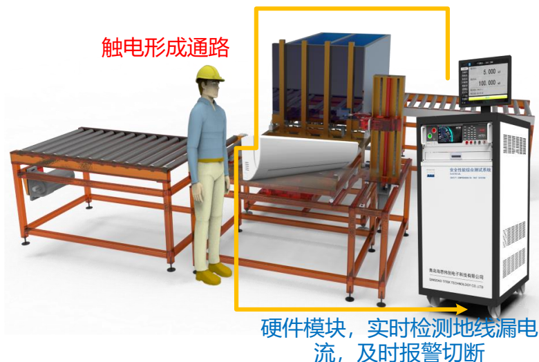
图 3-1-1 漏电快速断电保护原理
