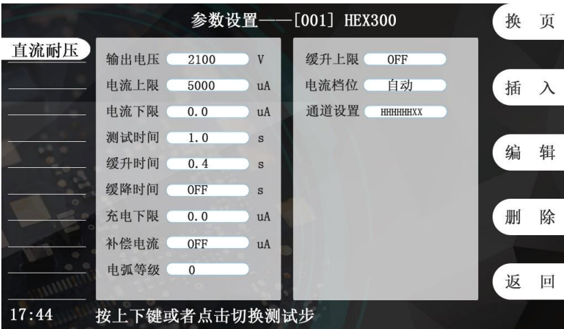
图 5-5-3 直流耐压设置界面
