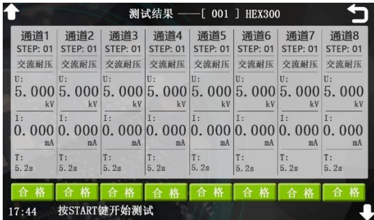
图 5-6-3 测试项全合格
