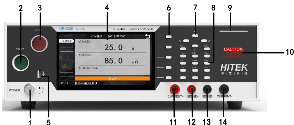
图 3-3-1 HEX303 前面板说明
