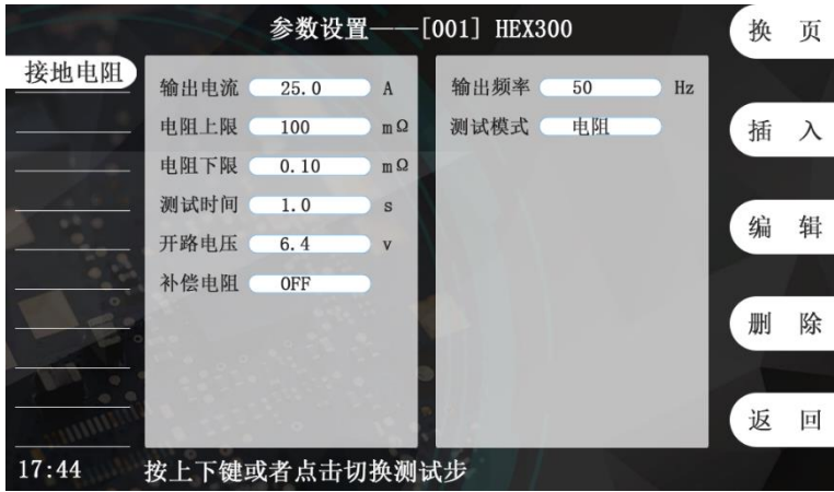
图 4-5-3 接地电阻设置界面
