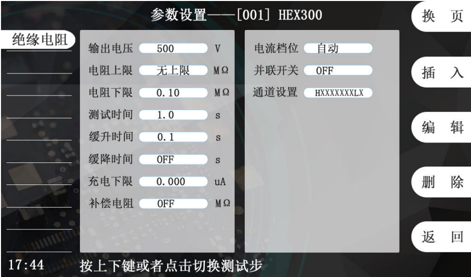
图 5-5-4 绝缘电阻设置界面
