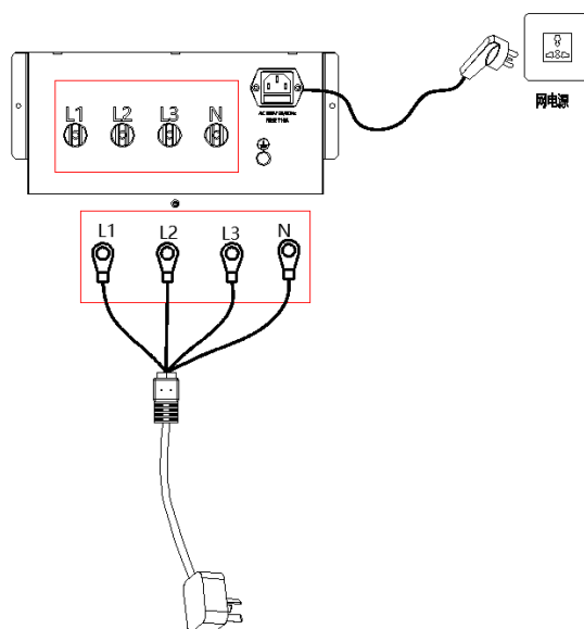
图 4-4-3 HEX440TM 连接本机电源
