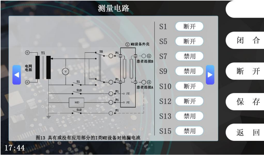
图 5-5-9 图 13 电路设置
