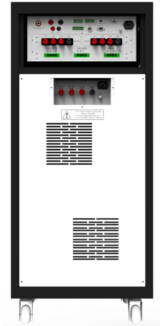
图 4-3-4 HEX440TM 背板
