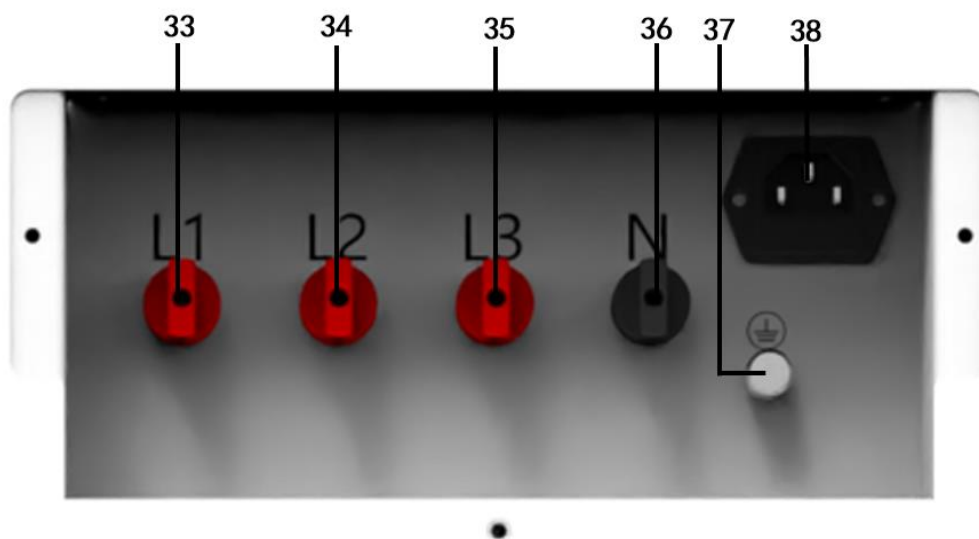
图 4-3-6 HEX440TM 背板放大图 2
