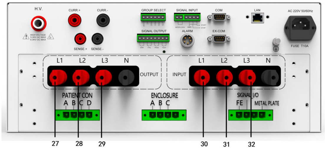
图 4-3-5 HEX440TM 背板放大图 1
