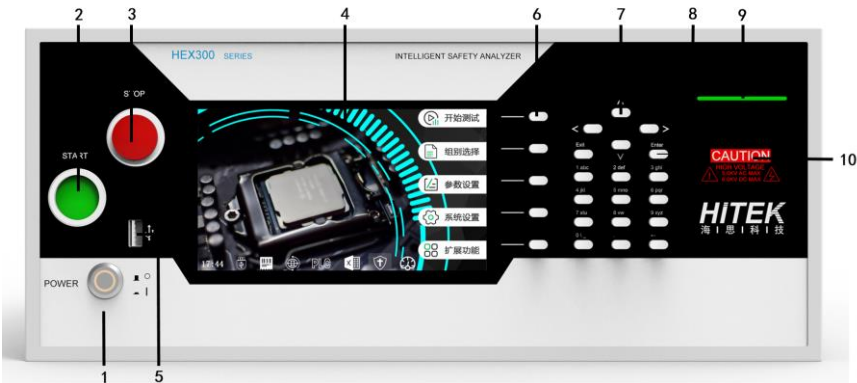
图 4-2-2 HEX440 系列前面板放大图
