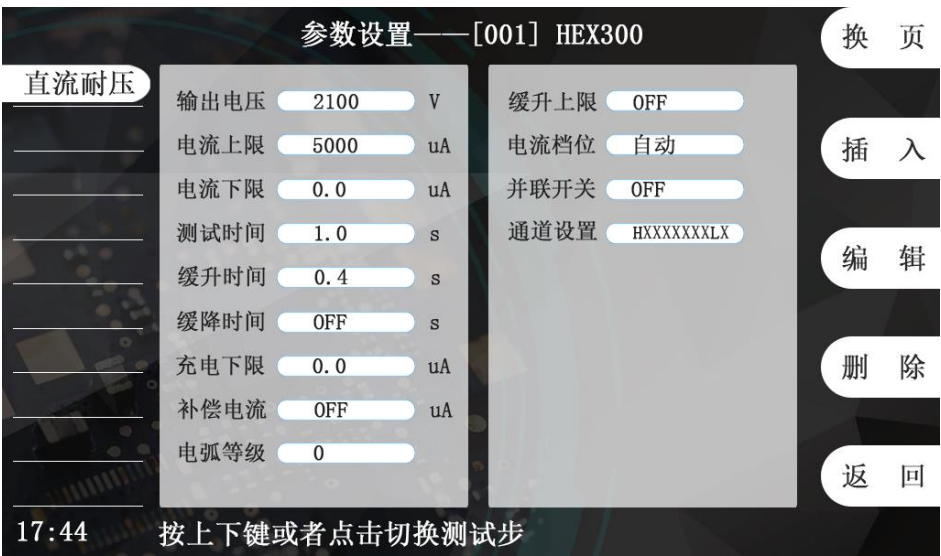
图 5-5-3 直流耐压设置界面
