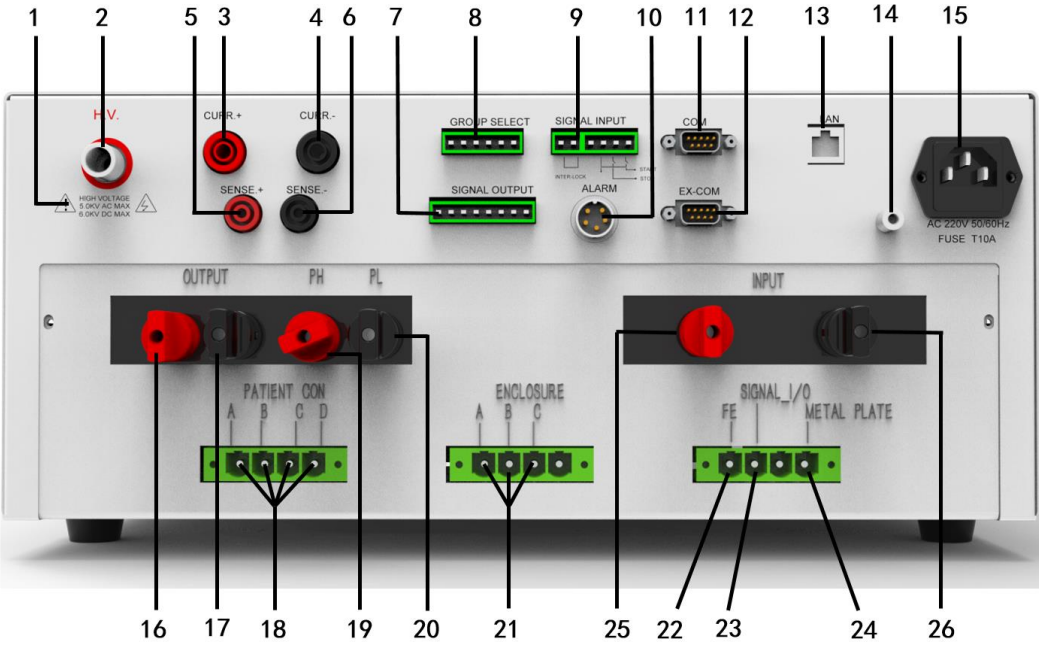
图 4-3-2 HEX440/HEX440M 背板放大图 1
