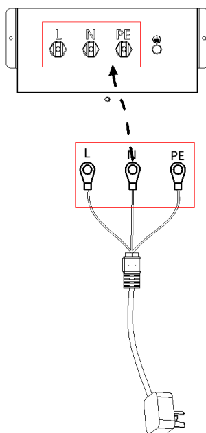
图 4-4-2 HEX440/HEX440M 连接本机电源
