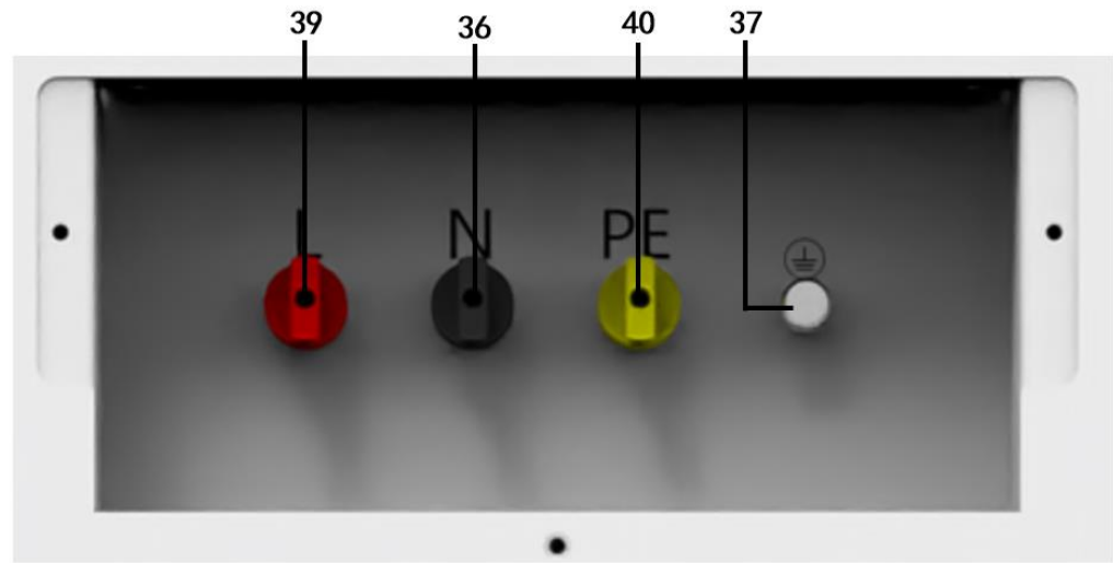
图 4-3-3 HEX440/HEX440M 背板放大图 2
