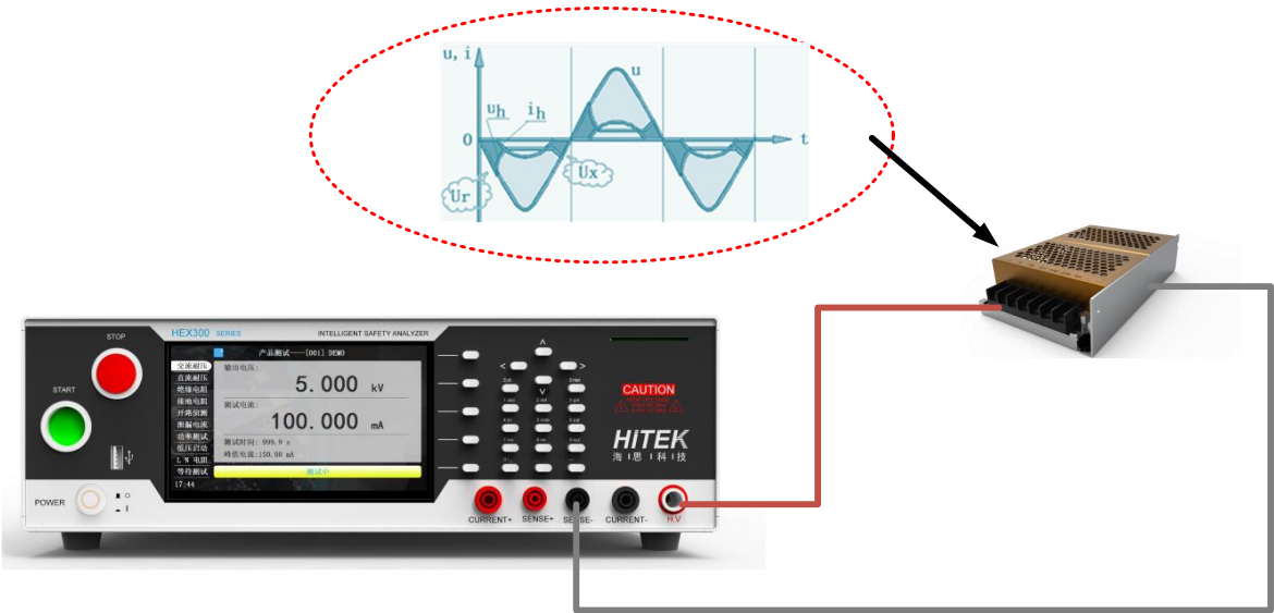
图 3-1-5 电弧侦测
