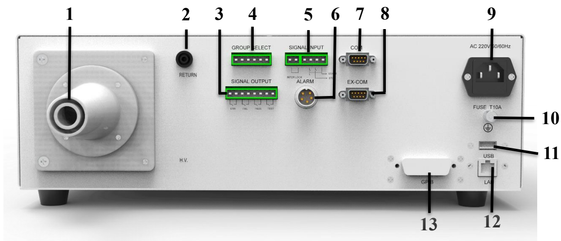
图 4-3-2 HEX3015/HEX3020 背板说明
