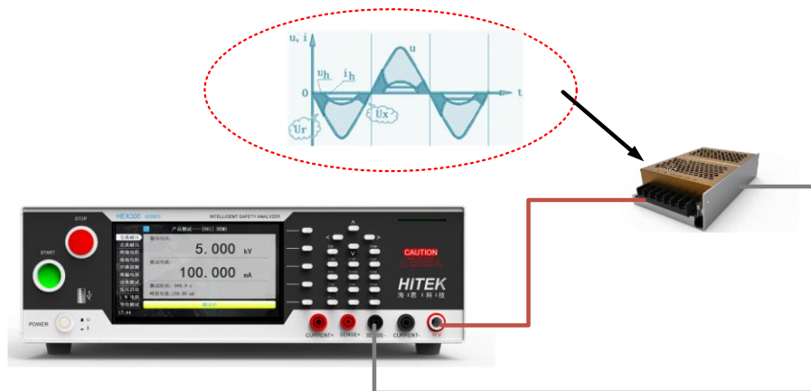
图 3-1-3 电弧侦测
