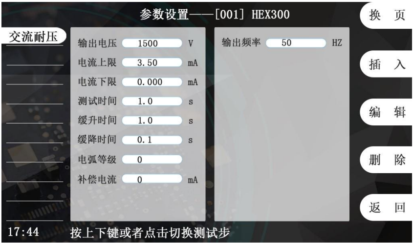
图 5-5-2 交流耐压设置界面
