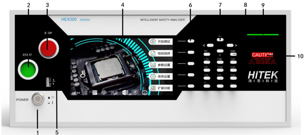
图 4-2-1 前面板说明
