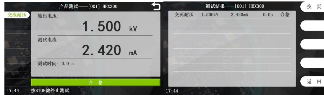
图 5-3-4 测试完成后显示单步结果
