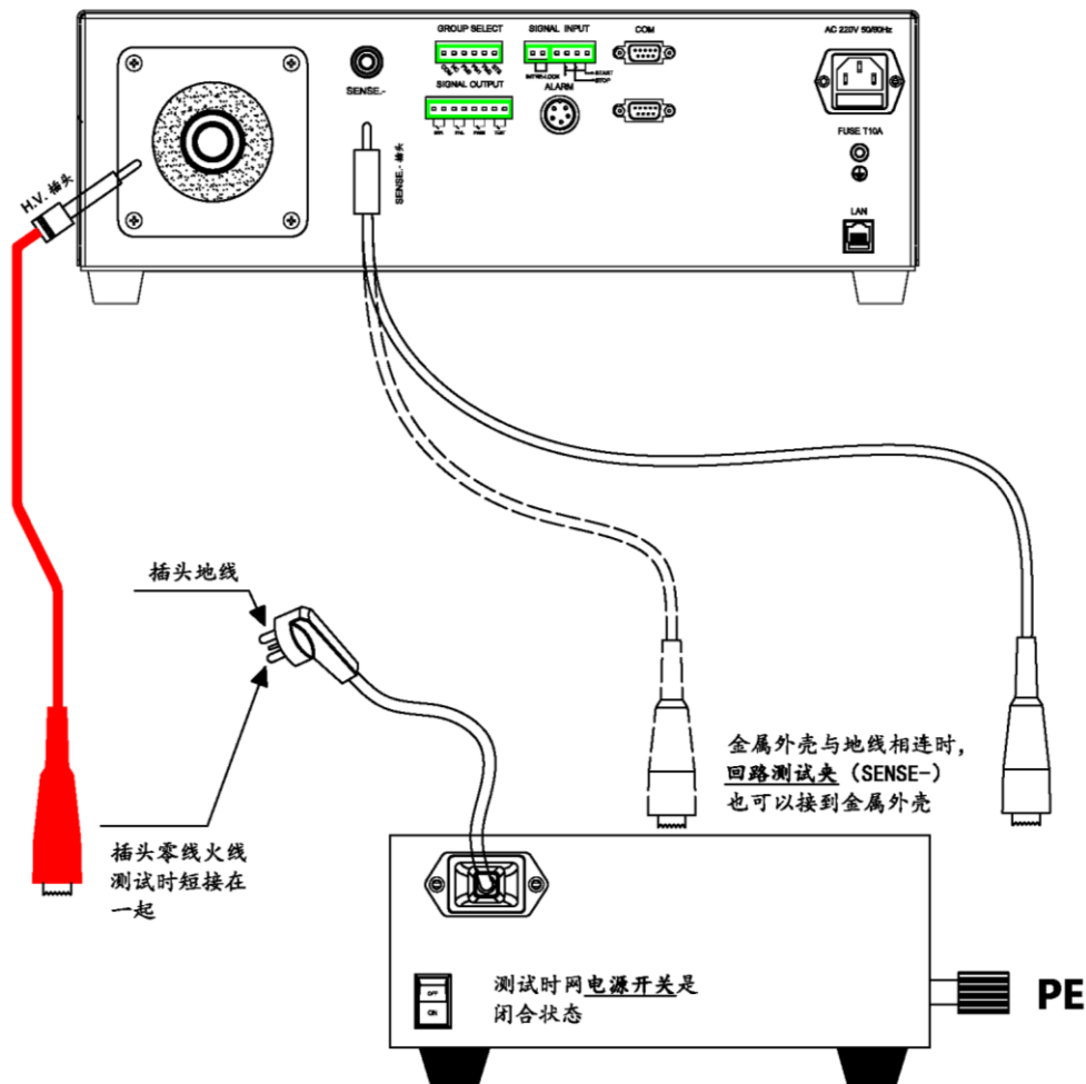
图 5-1-1 连接测试盒和回路测试夹示意图
