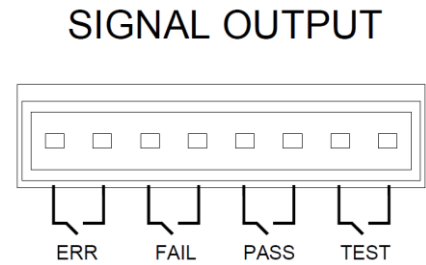
图 6-2-1 PLC 接口插座（公）
