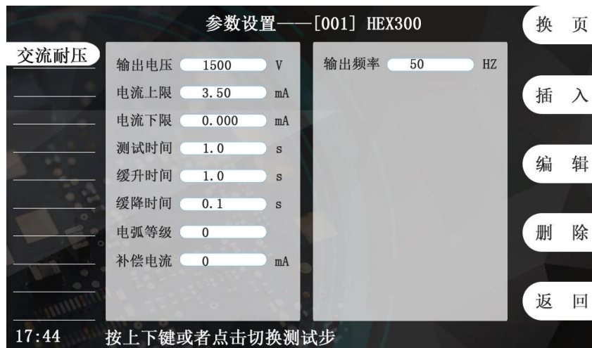
图 5-5-1 测试组设置界面
